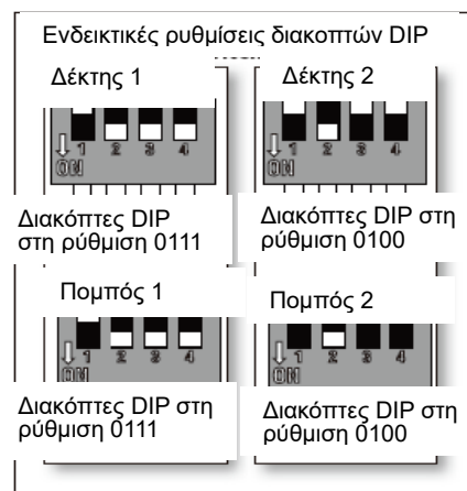
Εικ. 12 Διακόπτες DIP δέκτη
