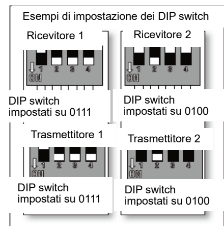
Fig. 12 DIP switch del ricevitore
