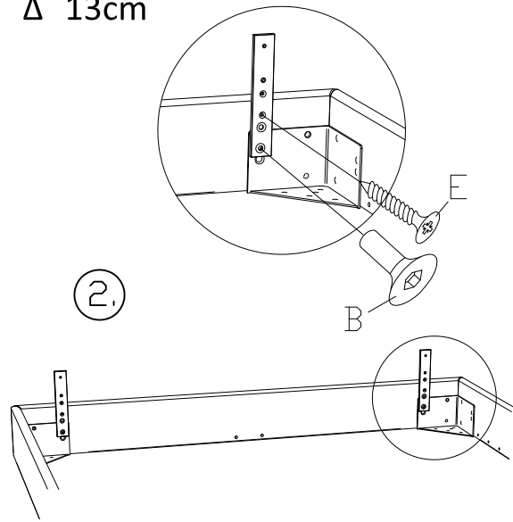
Variante B \Delta 13cm
